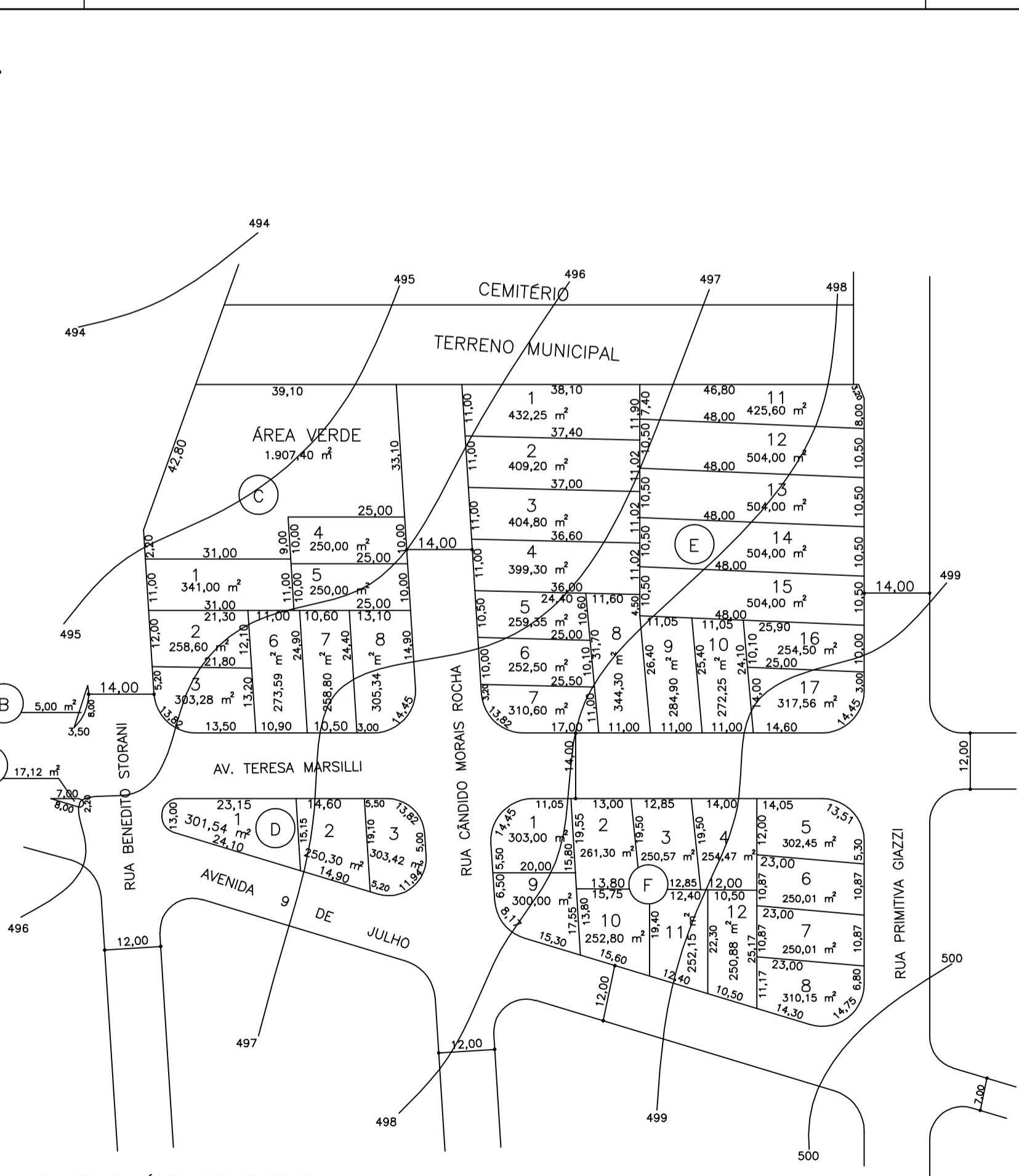
PLANTA DA ÁREA DESMEMBRADA ESCALA 1:1000
