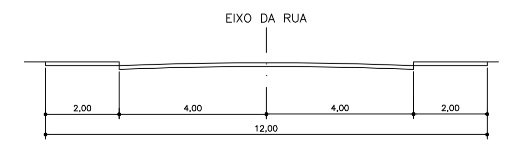
PERFIL TRANSVERSAL DAS VIAS ESCALA 1:100
